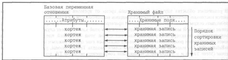
Рис. А.1. Реализация с прямым отображением
