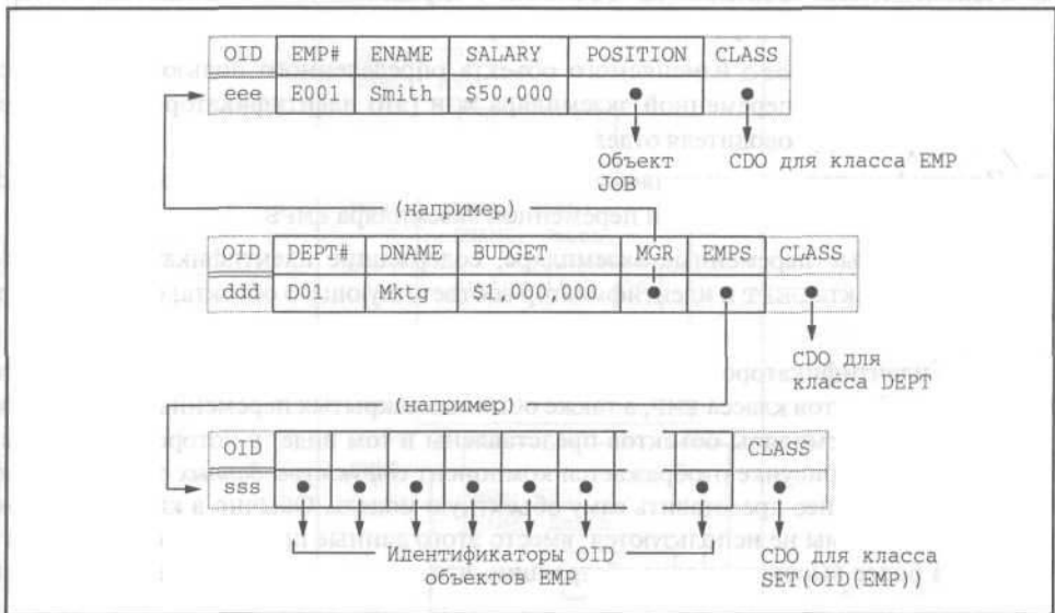
Рис. 25.4. Пример экземпляров объектов классов DEPT и EMP
