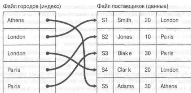
Рис. Г.9. Индексация файла поставщиков по атрибуту CITY
