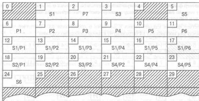
Рис. Г.3. Компоновка диска после вставки записи поставщика S6, удаления записи поставщика S2, вставки записи детали P7 и удаления записи поставщика S4
