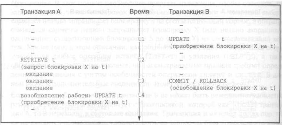
Рис. 16.8. Пример того, что для транзакции А исключена возможность обновлять незафиксированное изменение в момент времени t_2
