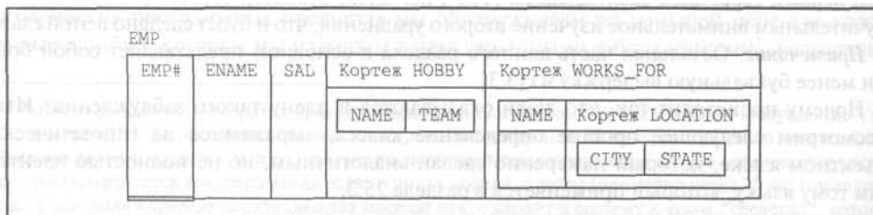
Рис. 26.1. Атрибуты, содержащие кортежи (указатели на кортежи). —
