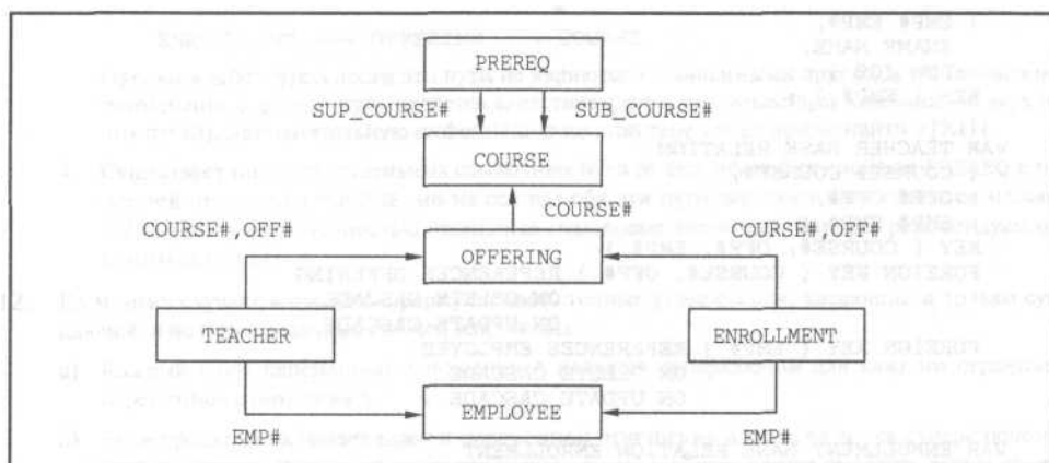
Рис. Д.5. Ссылочная диаграмма
