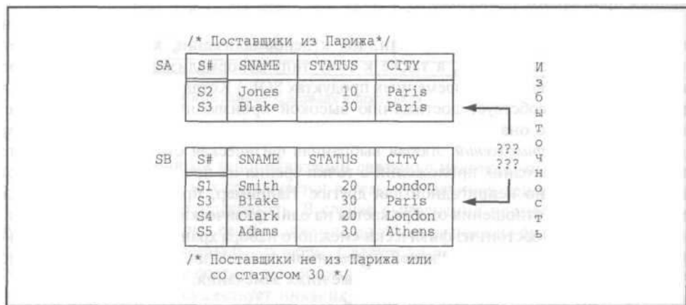
Рис. 13.7. Плохой, но вполне допустимый проект представления данных о поставщиках
