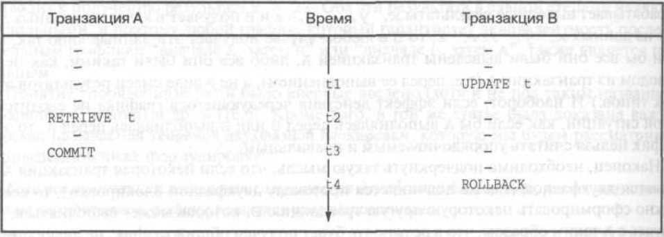
Рис. 16.11. Пример невозстановимого графика
