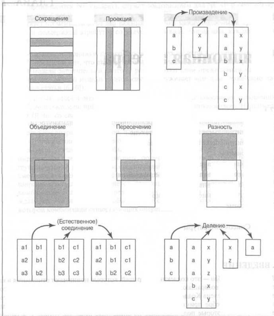
Рис. 7.1. Восемь первоначальных операций (краткая иллюстрация)
