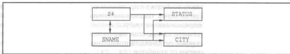
Рис. 12.12. Диаграмма функциональных зависимостей в переменной отношения S для случая, когда множество атрибутов {SNAME} является ее потенциальным ключом (и зависимость CITY → STATUS не выполняется)
