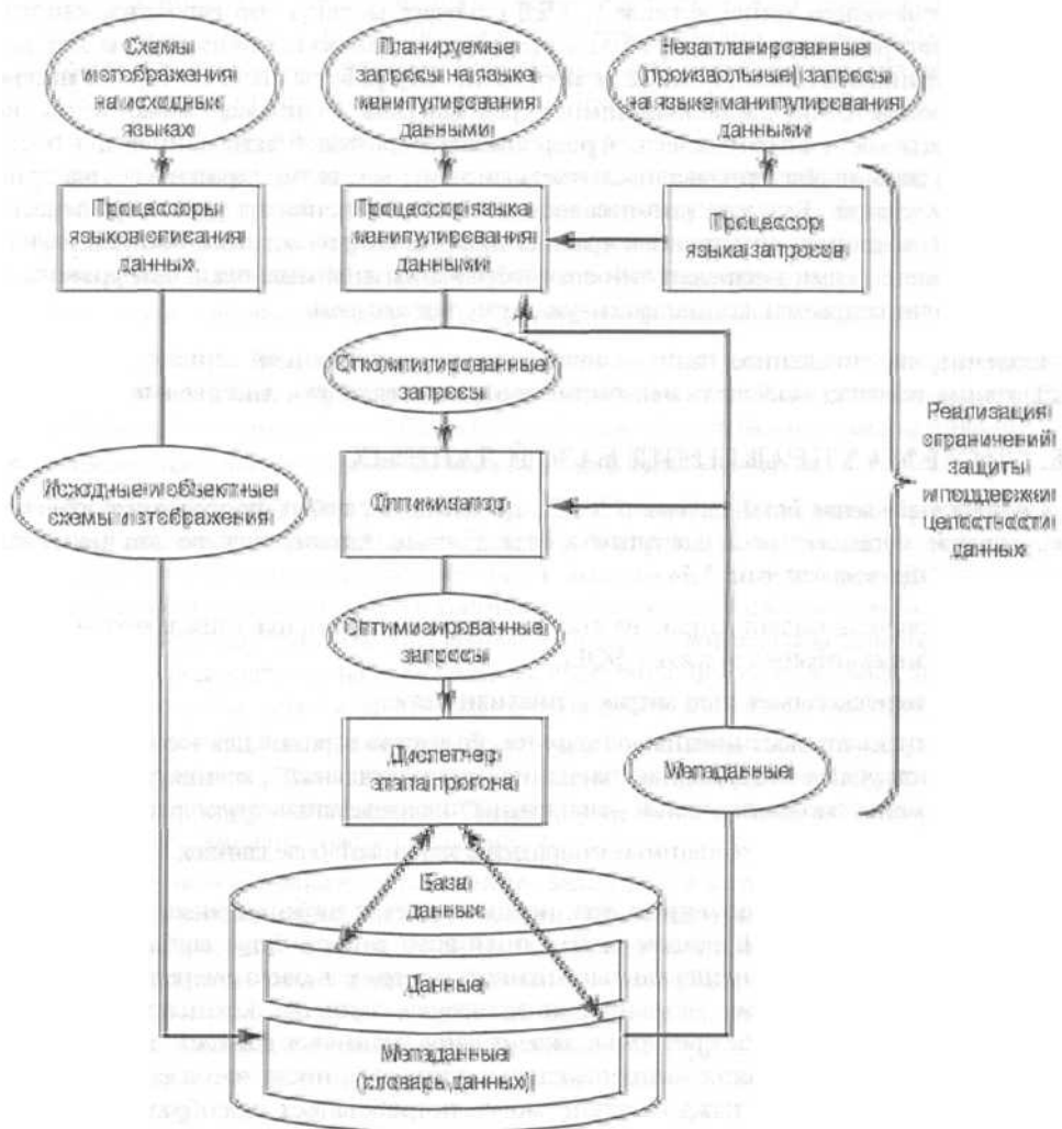
Рис. 2.4. Основные функции и компоненты типичной СУБД
